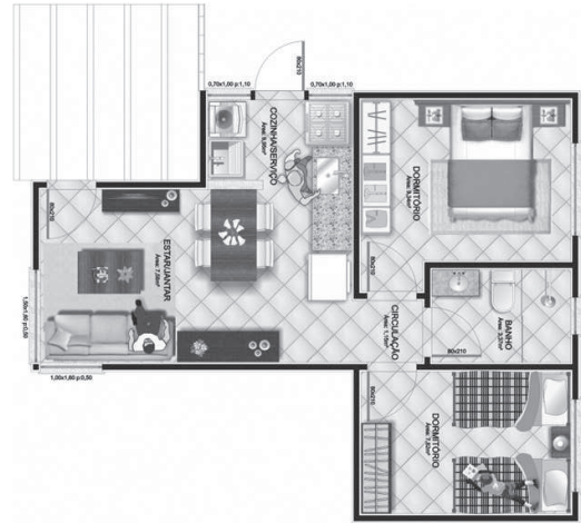
FIGURA 1 – Projeto base da Habitação de Interesse Social.
